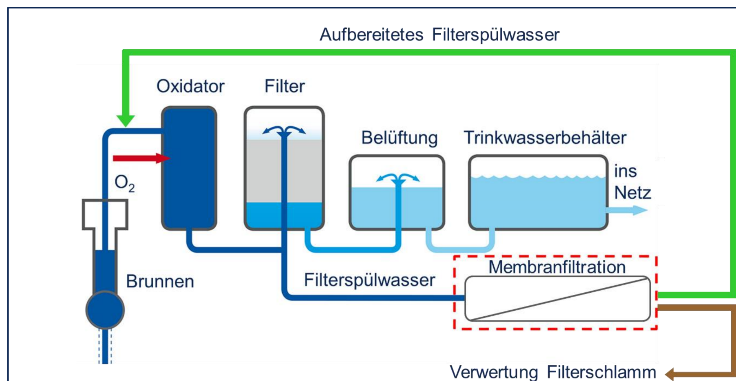
Schema der Trinkwasseraufbereitung mit untersuchter Option der Wiederverwendung
